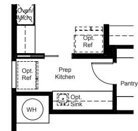
Optional Pantry Door
