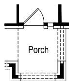
Opt 42" Door @ Entry
